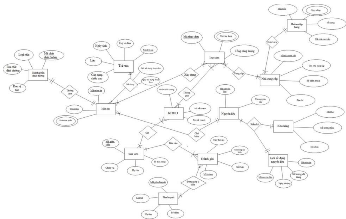
Hình 25. Mô hình thực thể liên kết ERM
