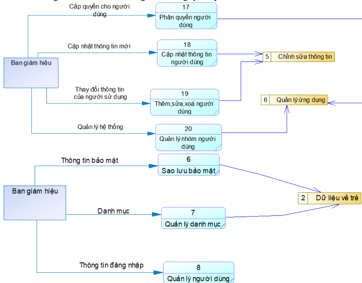
Hình 8. Biểu đồ mức 1- Chức năng Hệ thống quản lý
