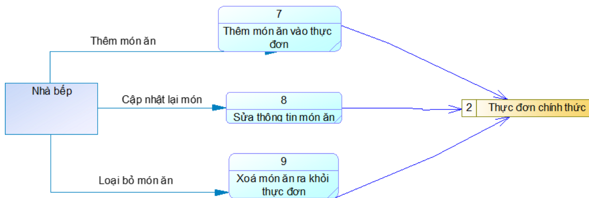
Hình 22. Biểu đồ mức 2 – Chức năng Cập nhật thực đơn
