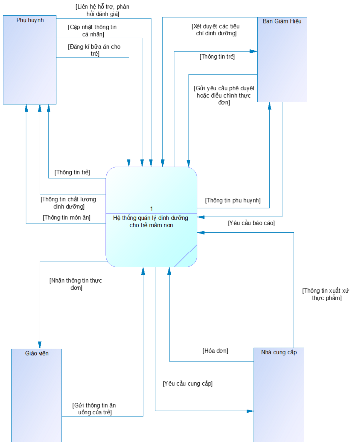
Hình 3. Biểu đồ ngữ cảnh
