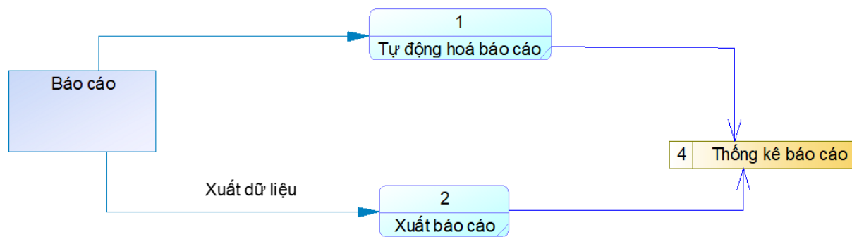
Hình 17. Biểu đồ mức 1-Chức năng Hệ thống báo cáo
