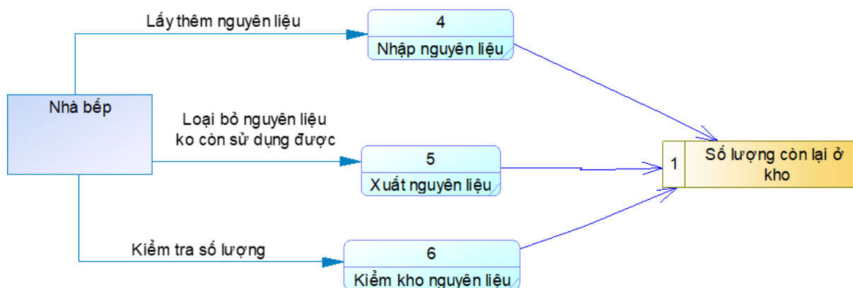
Hình 21. Biểu đồ mức 2 – Chức năng Xuất nhập nguyên liệu
