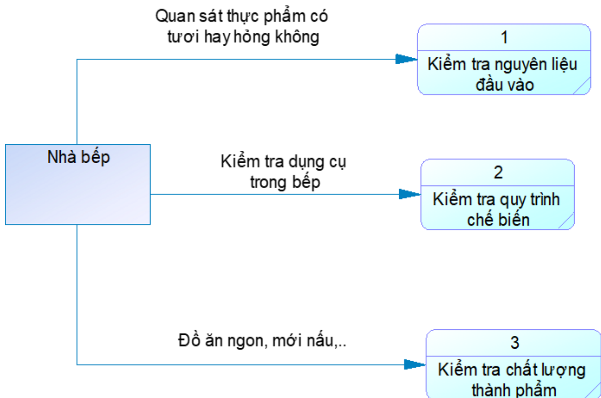
Hình 20. Biểu đồ mức 2 – Chức năng Kiểm tra chế biến
