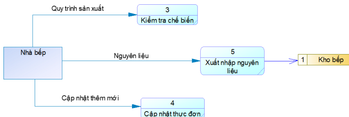
Hình 19. Biểu đồ mức 1-Chức năng Hệ thống nhà bếp
