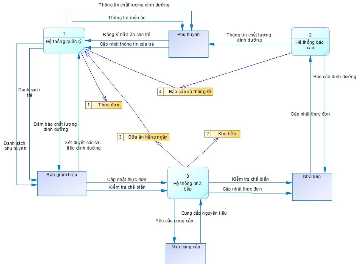
Hình 7. Biểu đồ mức 0
