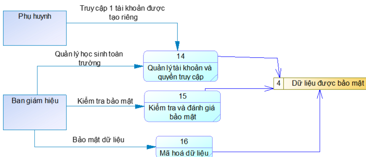
Hình 11. Biểu đồ mức 3 – Chức năng Bảo mật hệ thống
