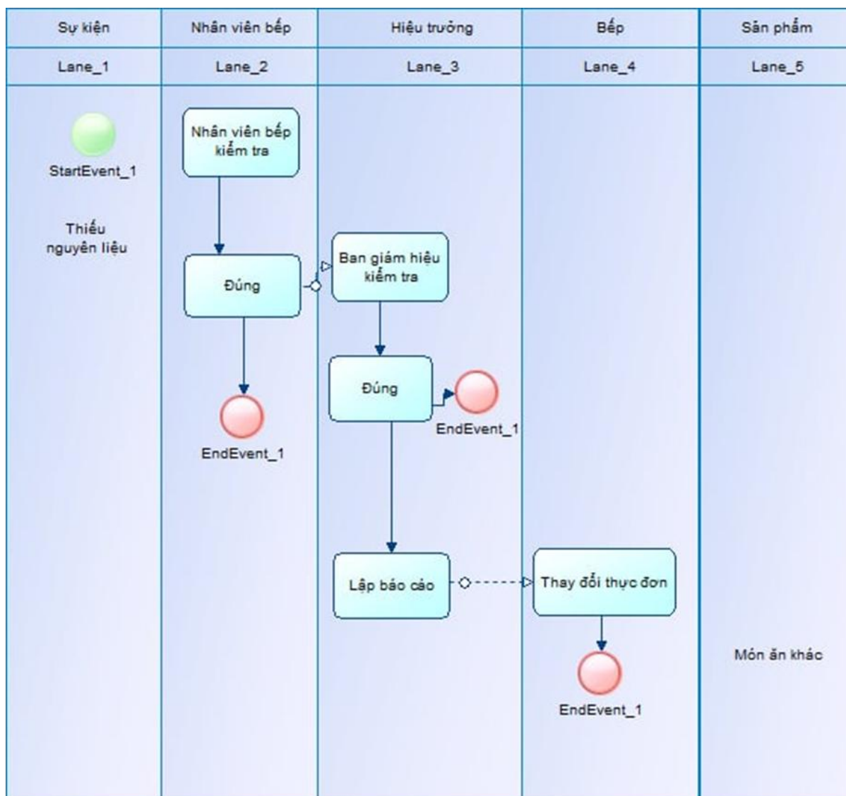
Hình 6. Biểu đồ hoạt động trường hợp “Thiếu nguyên liệu”
