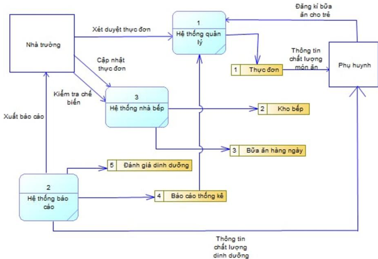
Hình 24. Biểu đồ luồng dữ liệu logic hệ thống quản lý dinh dưỡng cho trẻ mầm non
