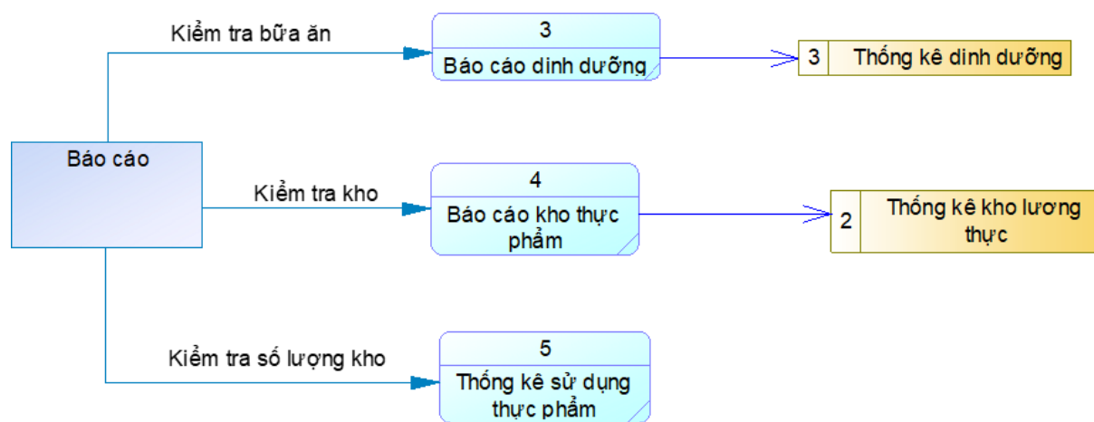
Hình 18. Biểu đồ mức 2-Chức năng Xuất báo cáo
