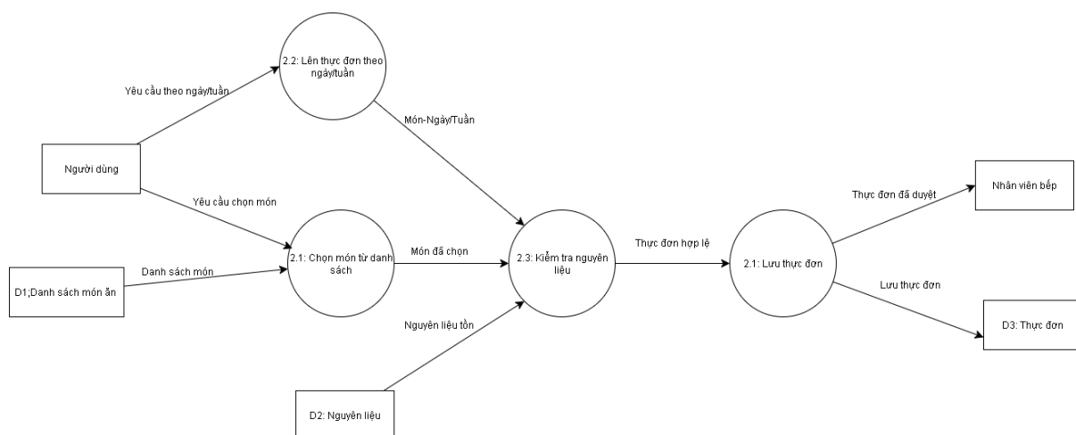
Hình 23. Biểu đồ mức 2 – Chức năng Lên thực đơn
