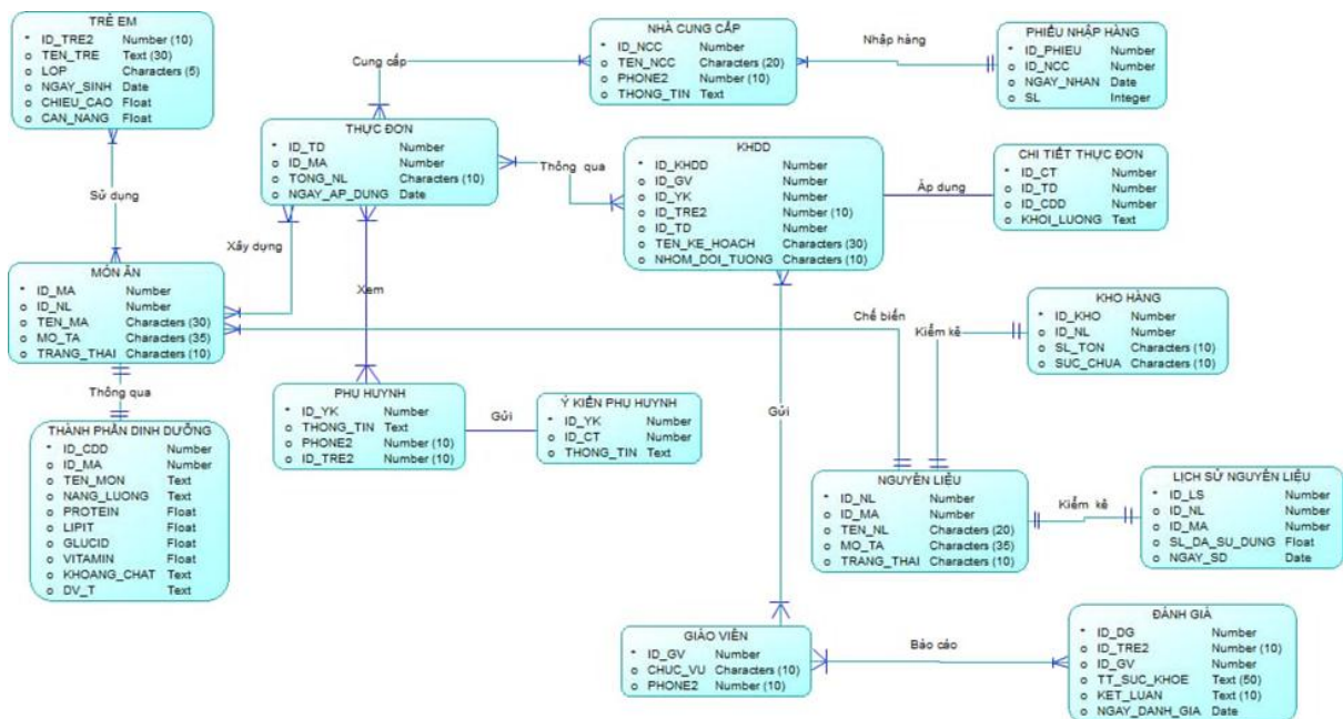
Hình 26. Mô hình quan hệ
