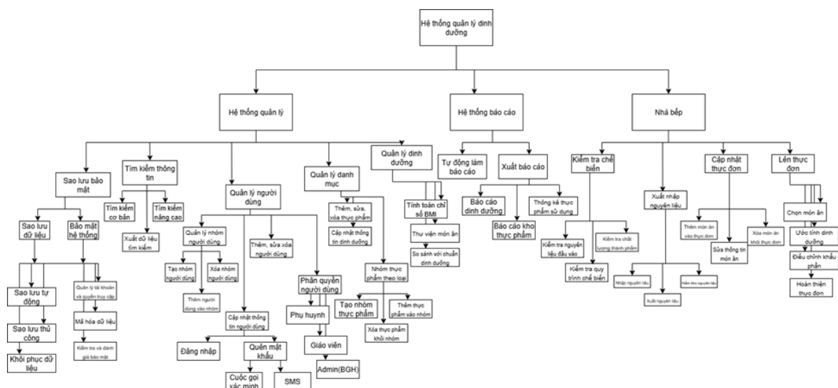
Hình 4. Biểu đồ phân rã chức năng
