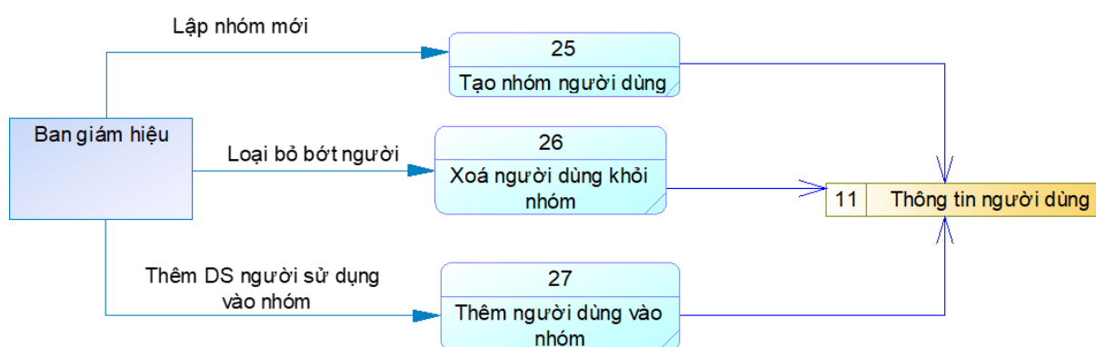
Hình 16. Biểu đồ mức 3- Chức năng Quản lý nhóm người dùng
