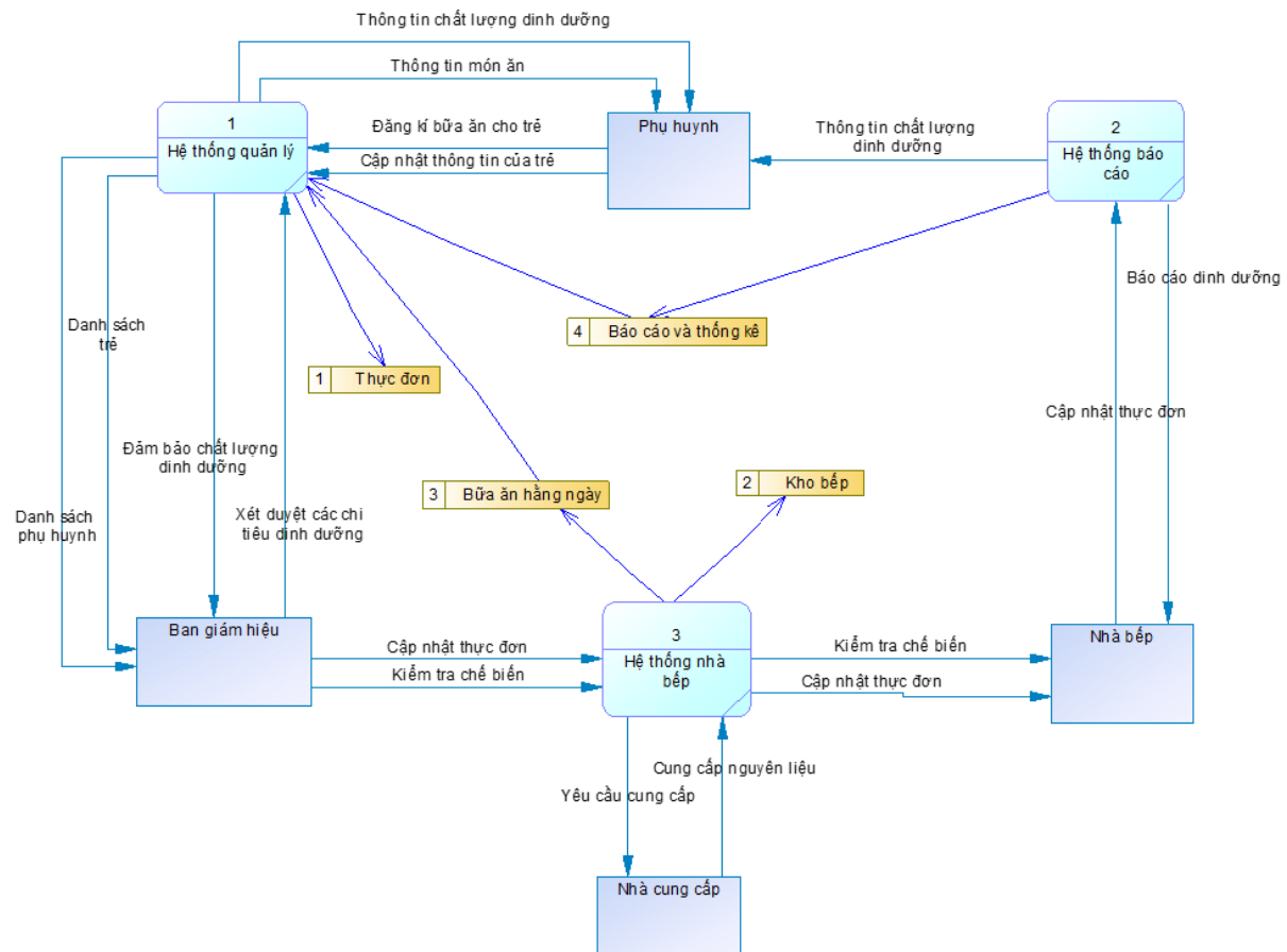
Hình 24. Biểu đồ luồng dữ liệu vật lý của hệ thống quản lý dinh dưỡng cho trẻ mầm non
