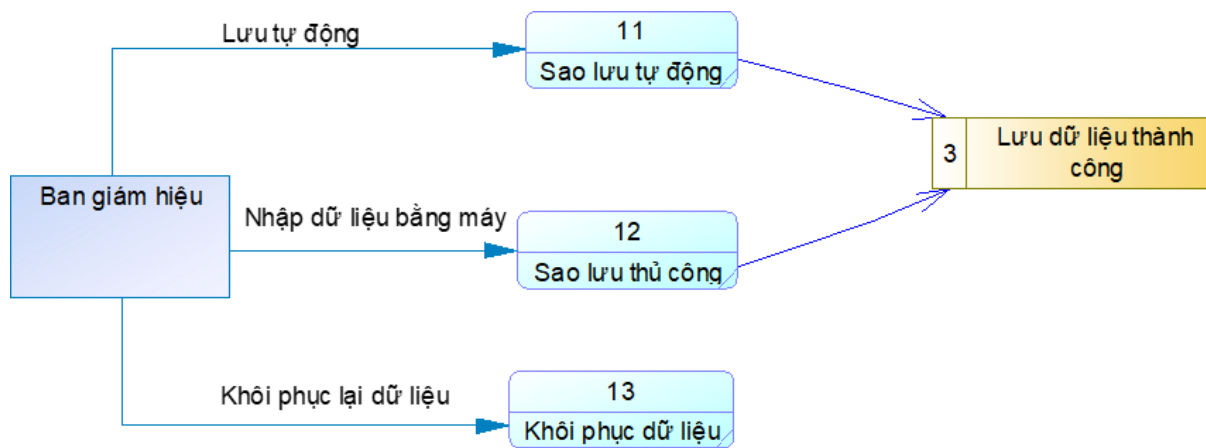
Hình 10. Biểu đồ mức 3 – Chức năng Sao lưu dữ liệu
